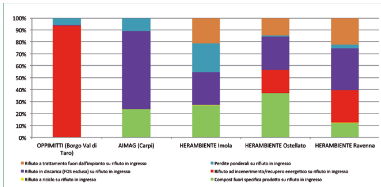
Figura 1.26> Bilancio di massa degli impianti TMB, 2015
