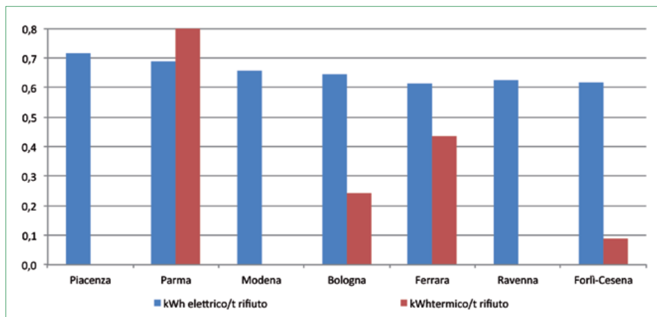
Figura 1.27> Impianti di incenerimento: kWh prodotti su tonnellata di rifiuto incenerito, 2015
