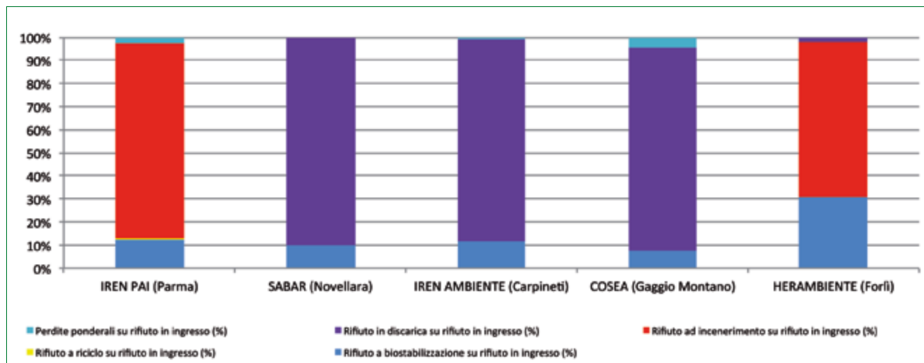
Figura 1.25> Bilancio di massa degli impianti TM, 2015
