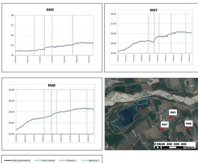
Fig. 7 - Andamento del livello piezometrico in 3 punti lontani dal lago di ricarica.
