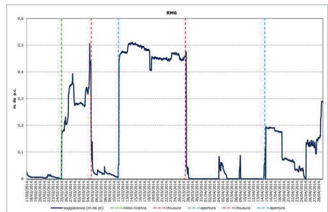
Fig. 5 - Livello idrometrico del canale di adduzione al lago di ricarica.
