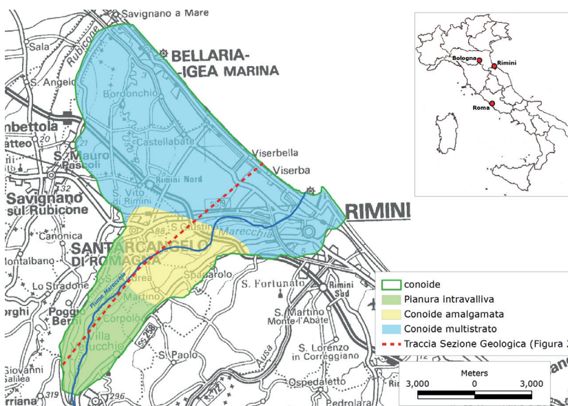
Fig. 1 - Conoide del Fiume Marecchia e suoi diversi ambiti (pianura intravalliva, conoide amalgamata e conoide multistrato).
