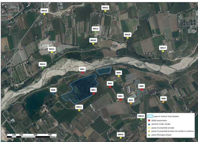
Fig. 4 - Rete di monitoraggio per la verifica dell'efficacia dell'intervento di ricarica in condizioni controllate.
