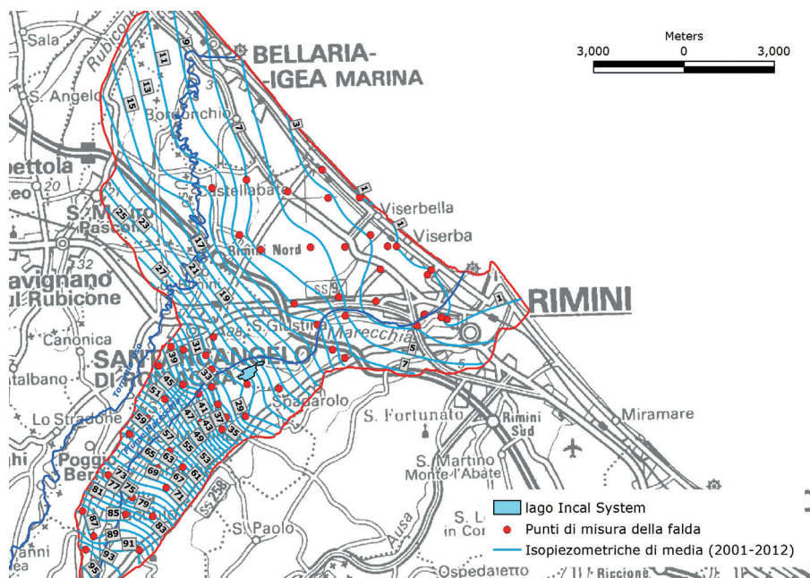
Fig. 3 - Superficie piezometrica media della conoide del Marecchia (2001-2012).
