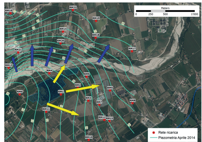
Fig. 8 - Piezometria nelle vicinanze del lago di ricarica nell'Aprile 2014. Le frecce gialle indicano il flusso dal lago di ricarica alla conoide, quelle blu il flusso verso il Fiume Marecchia e la parte nord della conoide.
