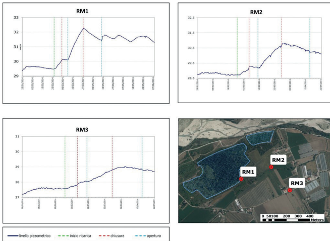
Fig. 6 - Andamento del livello piezometrico in 3 punti vicini al lago di ricarica.
