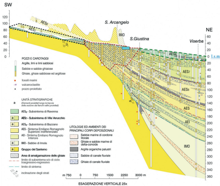
Fig. 2 - Sezione geologica longitudinale della Conoide del Marecchia con schematizzazione degli acquiferi e ubicazione del lago di ricarica Incal System (box azzurro). Sono indicate la piana intravalliva (area con tratteggio nero); la conoide amalgamata (area con tratteggio rosso), la conoide multistrato (a valle delle precedenti) e l'acquifero freatico di pianura (area con tratteggio verde), (da Servizio Geologico d'Italia – Regione Emilia-Romagna 2005, modificata).
