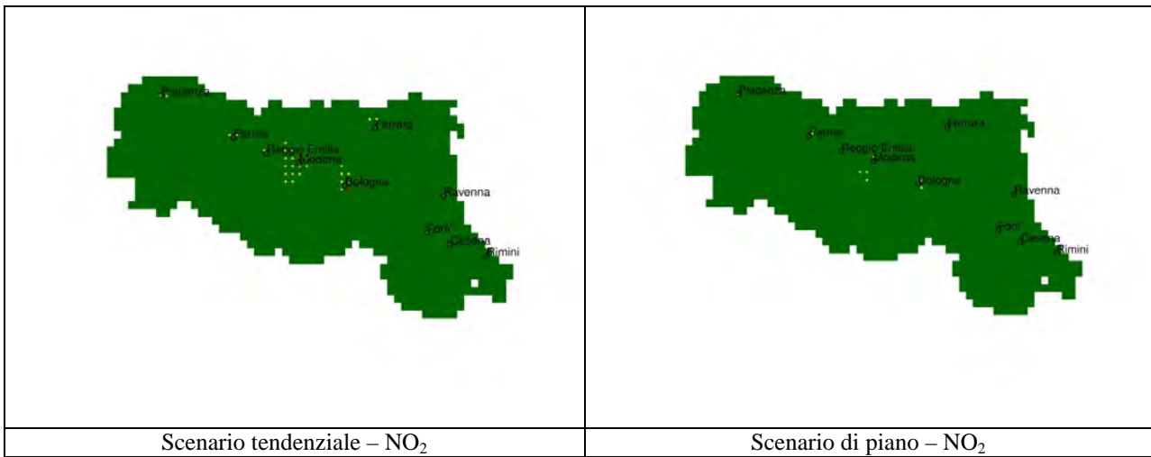
Figura 10.2.2 - Aree di superamento del VL annuale per NO 2 nello scenario di piano. Superamenti su tutto il territorio in tutti gli anni (aree con colorazione rossa continua), Superamenti su parte del territorio in tutti gli anni (aree con colorazione gialla con puntini rossi), Superamenti su tutto il territorio in alcuni anni (aree con colorazione gialla continua), Superamenti su parte del territorio in alcuni anni (aree con colorazione verde con puntini gialli), Non si verificano superamenti (aree con colorazione verde continua). Scenario tendenziale a sinistra, scenario di piano a destra.
