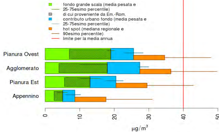
Figura 5.3.4 - Origine geografica dell'inquinamento da NOx
