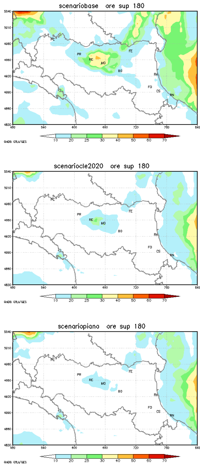
Figura 10.2.4 - Numero di ore di superamento della soglia di formazione (valore orario superiore a 180 •g/m 3 ) nello scenario di riferimento (in alto), nello scenario tendenziale (al centro) e nello scenario di piano (in basso)
