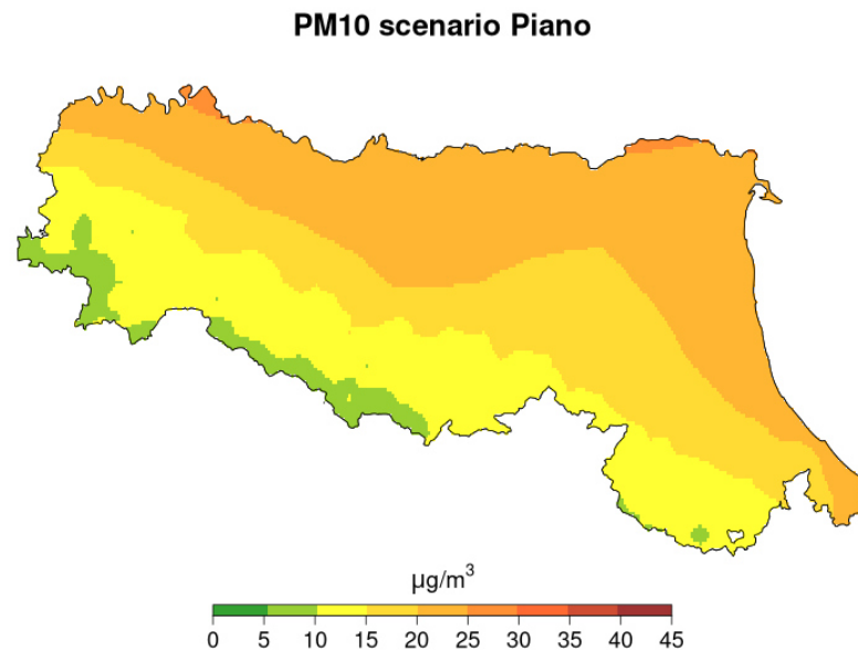
Fig. 99: Concentrazioni medie annuali di PM10 (µg/m 3 ) dello scenario di piano
