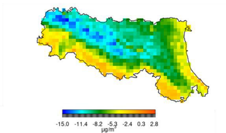
Fig. 106: Differenze del 93.2° percentile della massima concentrazione giornaliera delle media mobile su 8 ore di ozono tra lo scenario di piano e lo scenario base
