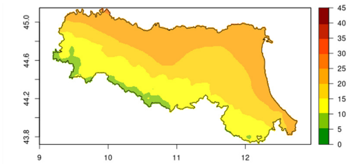
Fig. 52: Media annuale di PM10 ( \mu\text{g}/\text{m}^3 ), scenario teorico
