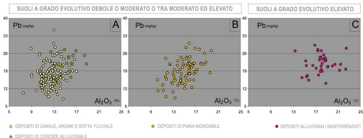
Figura 12. Diagramma Pb/Al_2O_3 relativo a suoli a diversa granulometria e differente grado evolutivo.
