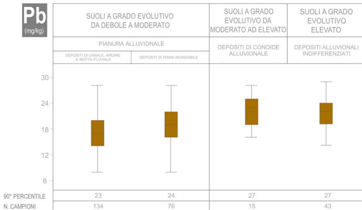
Figura 13. Caratterizzazione geochimica dei suoli della pianura emiliana relativamente al contenuto pedo-geochimico in Pb. Il tenore naturale di Pb nei suoli è principalmente funzione del grado evolutivo: si osserva un relativo arricchimento nei suoli da moderata ad elevata differenziazione del profilo.
