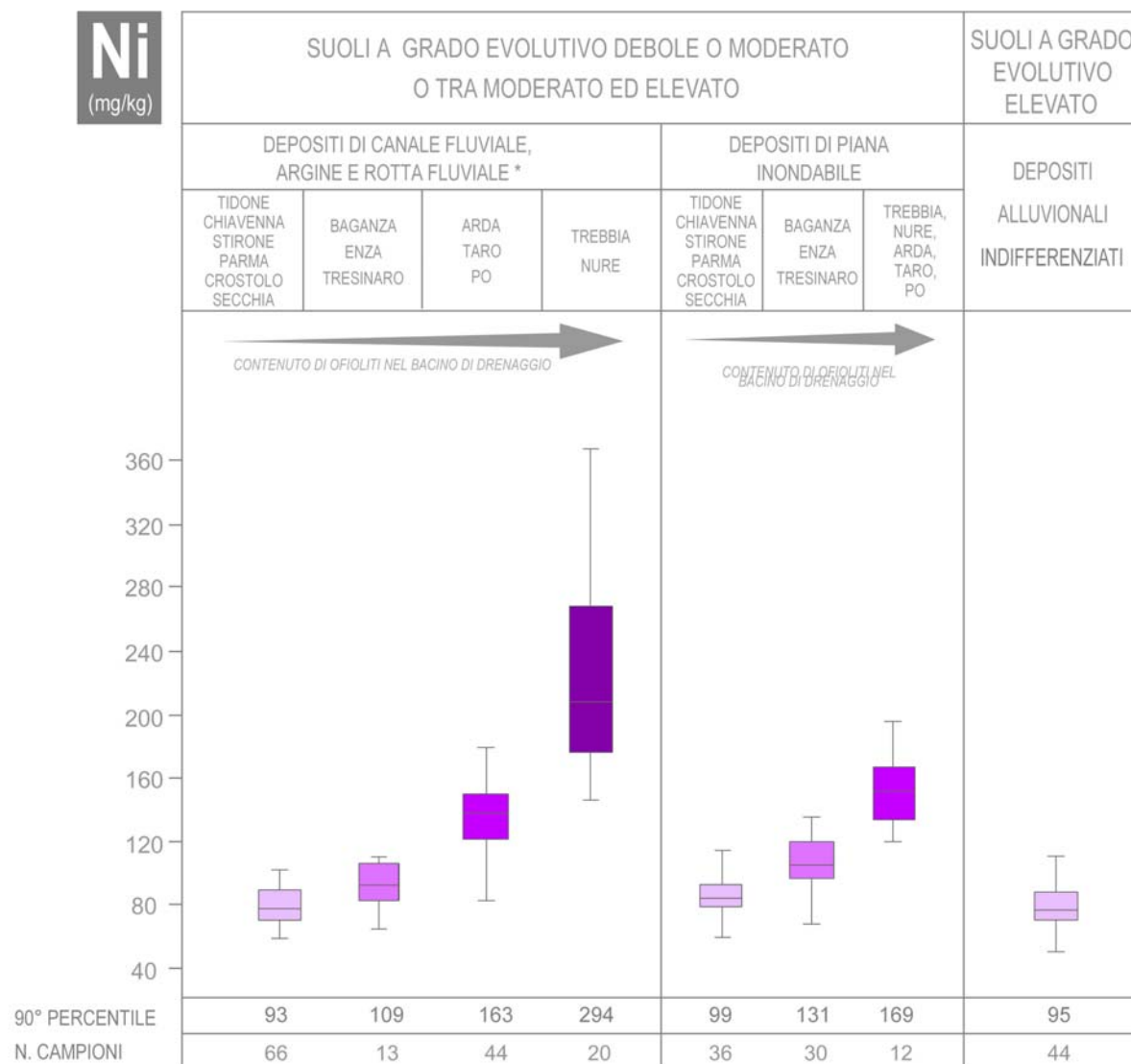
Figura 4. Caratterizzazione geochemica dei suoli della pianura emiliana relativamente al contenuto pedo-geochemico in Ni. I suoli sono distinti in primo luogo sulla base del grado evolutivo. Un secondo livello classificativo distingue le due principali associazioni di facies (canale, argine e rotta fluviale vs piana inondabile) dei sistemi di pianura alluvionale e conoide analizzate per domini di provenienza. I dati sono rappresentati per valori crescenti del contenuto di ofioliti all'interno dei bacini di drenaggio. Al di sotto di ogni box plot viene riportato il valore di concentrazione di metallo relativo al 90° percentile, nonché il numero di campioni "N" utilizzati per la costruzione del box-plot. Si osservi il comportamento di Ni, analogo rispetto a Cr sia per quanto concerne la distribuzione in base alla provenienza del sedimento, che per quanto riguarda il preferenziale accumulo di metallo all'interno dei sedimenti fini.
