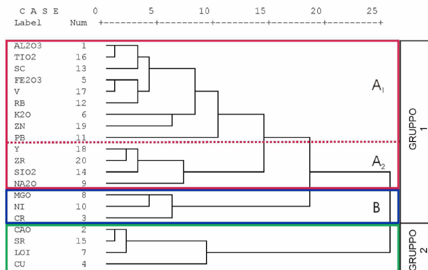
Figura 16. Dendrogramma delle variabili ottenuto dall'analisi cluster.
