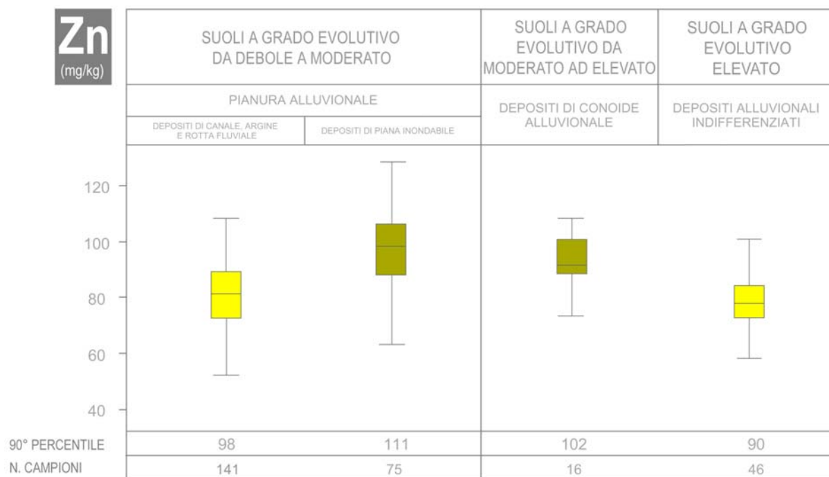
Figura 7. Caratterizzazione geochimica dei suoli della pianura emiliana relativamente al contenuto pedo-geochimico in Zn. Il tenore naturale di Zn nei suoli è principalmente funzione della granulometria: si osserva un relativo accumulo del metallo all'interno delle argille e dei limi di piana inondabile e dei sedimenti siltoso-argillosi che chiudono al tetto sedimenti di conoide alluvionale.
