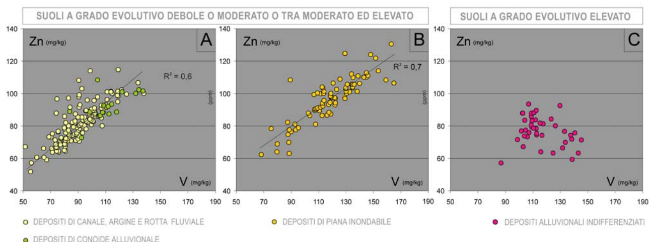
Figura 6. Diagramma Zn/V relativo a suoli a diversa granulometria e differente grado evolutivo.
