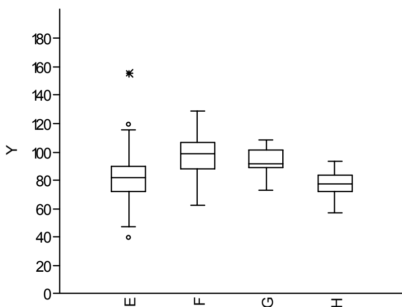
Figura 18. Esempio di box-plot con individuazione degli outliers relativi allo Zinco.
