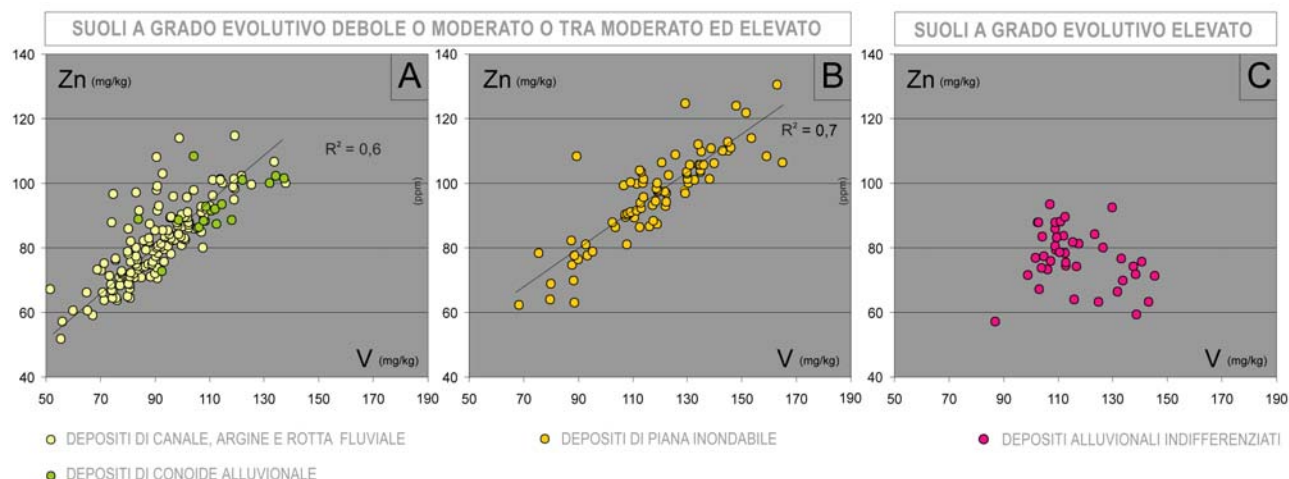
Figura 17. Diagramma Zn/V relativo a suoli a diversa granulometria e differente grado evolutivo.
