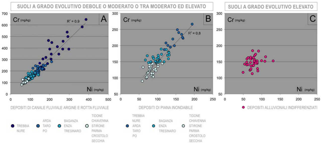
Figura 1. La provenienza di Cr e Ni da una stessa area fonte, così come l'appartenenza di questi due elementi alle stesse fasi mineralogiche, sono documentate nei suoli a debole/moderato e da moderato ad elevato grado evolutivo dai diagrammi A e B, che mostrano una forte correlazione positiva fra le due variabili, espressa da elevati valori di R^2 . I suoli nei depositi di canale, argine, rotta fluviale e conoide (A) e i suoli nei depositi di piana inondabile (B) mostrano tendenze analoghe. Lo stesso segnale non è chiaramente riconoscibile nei suoli ad elevata differenziazione del profilo (C).
