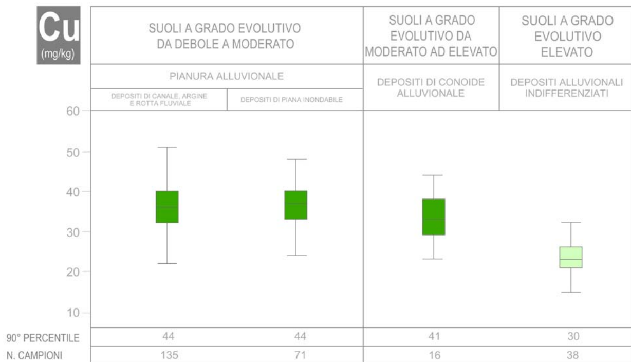
Figura 10. Caratterizzazione geochimica dei suoli della pianura emiliana relativamente al contenuto pedo-geochimico in Cu. Si noti come il tenore naturale di Cu nei suoli sia principalmente funzione del grado evolutivo, osservandosi un relativo impoverimento nei suoli ad elevata differenziazione del profilo
