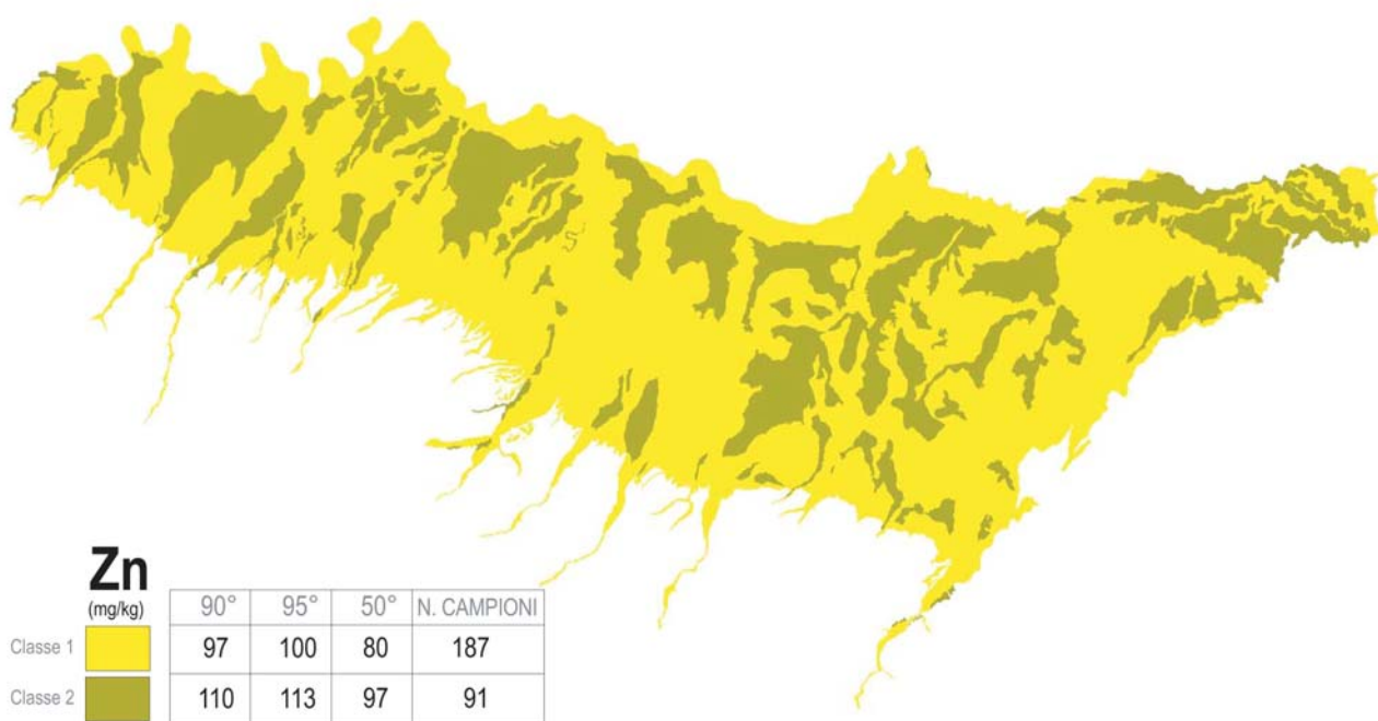
Figura 20. Carta pedo-geochemica di Zn della pianura emiliana.
