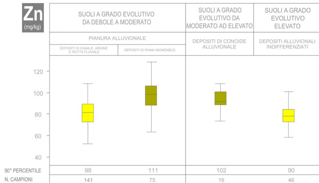
Figura 19. Caratterizzazione geochemica dei suoli della pianura emiliana relativamente al contenuto pedo-geochemico in Zn.
