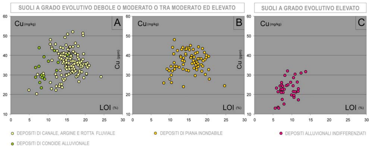
Figura 9. Diagrammi Cu/LOI (Loss on Ignition) relativo a suoli a diversa granulometria e differente grado evolutivo.
