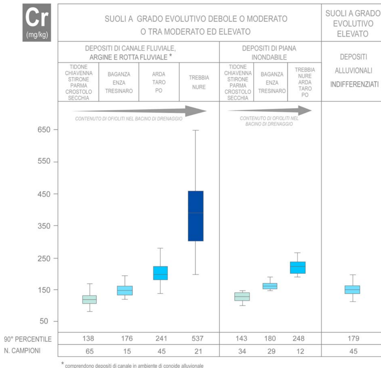
Figura 2. Caratterizzazione geochimica dei suoli della pianura emiliana relativamente al contenuto pedo-geochimico in Cr. I suoli sono distinti in primo luogo sulla base del grado evolutivo. Un secondo livello classificativo distingue le due principali associazioni di facies (canale, argine e rotta fluviale vs piana inondabile) dei sistemi di pianura alluvionale e conoide analizzate per domini di provenienza. I dati sono rappresentati per valori crescenti del contenuto di ofioliti all'interno dei bacini di drenaggio. Al di sotto di ogni box plot viene riportato il valore di concentrazione di metallo relativo al 90° percentile, nonché il numero di campioni "N" utilizzati per la costruzione del box-plot.
