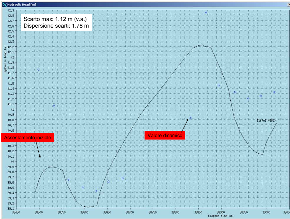
Pozzo Eiffel 685
