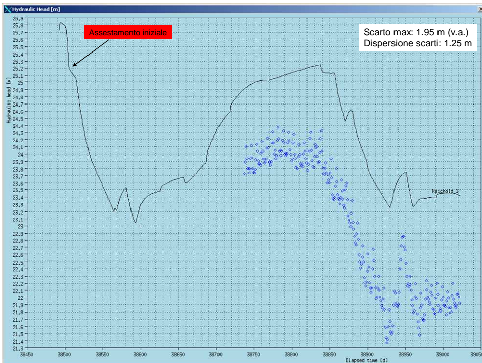
Pozzo Reichold 1
