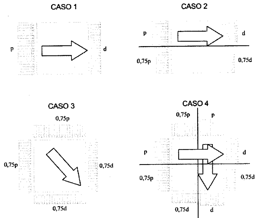
Figura 3.3.9 - Distribuzioni non simmetriche delle pressioni.
