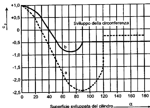
Figura 3.3.12 - Coefficienti di pressione esterna delle superfici cilindriche e sferiche: curva (a) per superfici lisce (metalliche, intonaco liscio); curva (b) per superfici ruvide (muratura con giunti di malta, intonaco rustico)
