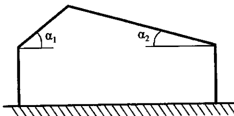
Figura 3.5.5 – Condizioni di carico per coperture a due falde
