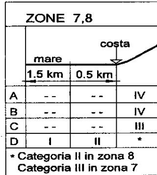
Figura 3.3.3 - Definizione delle categorie di esposizione I, II, III, IV e V, in funzione delle regioni individuate nella macrozonazione
