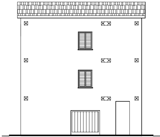
PROSPETTO FRONTE
