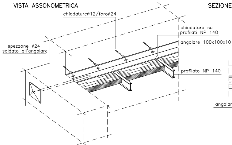
VISTA ASSONOMETRICA
