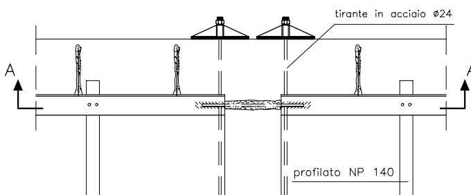
PIANTA
