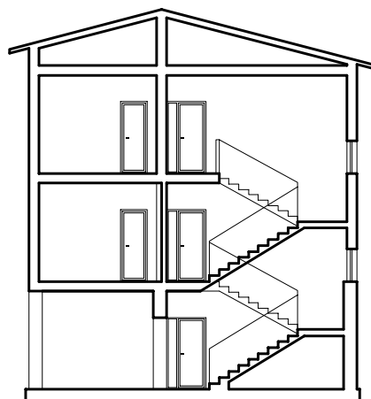
SEZIONE A:A
