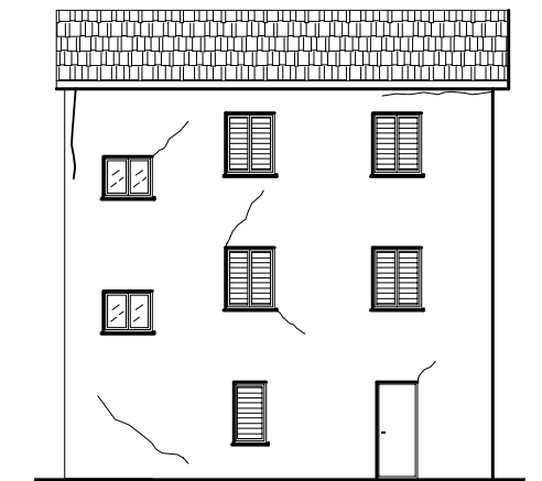
PROSPETTO RETRO
