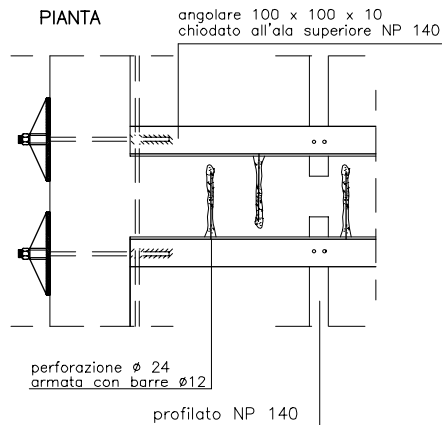
PARTICOLARE D
