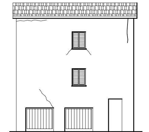
PROSPETTO FRONTE
