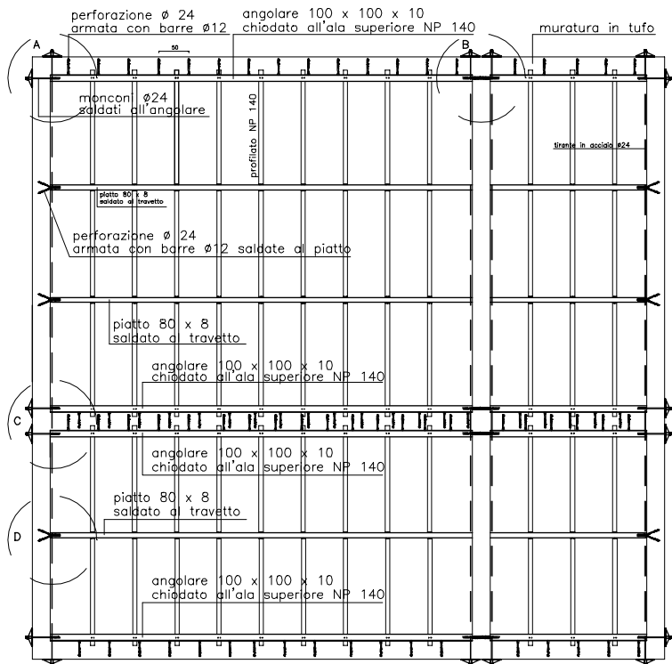
PIANTA
