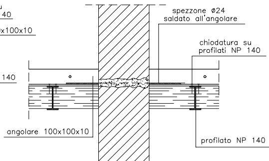
SEZIONE A-A
