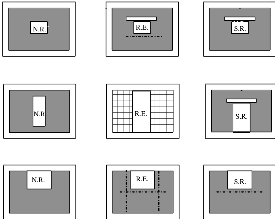
Figura 8.3: Schemi illustrativi delle condizioni di rinforzo delle aperture
