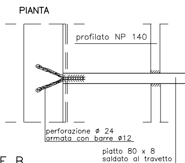
PARTICOLARE D
