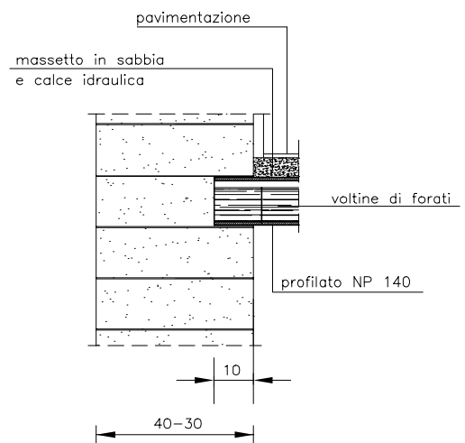
SEZIONE TRASVERSALE
