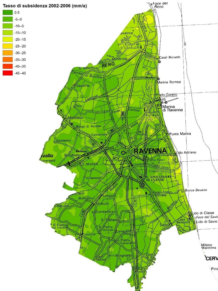
Fig. 2.2 – Tasso di subsidenza nel periodo 2002-2006 nell'area del Comune di Ravenna (Fonte ARPAE)
