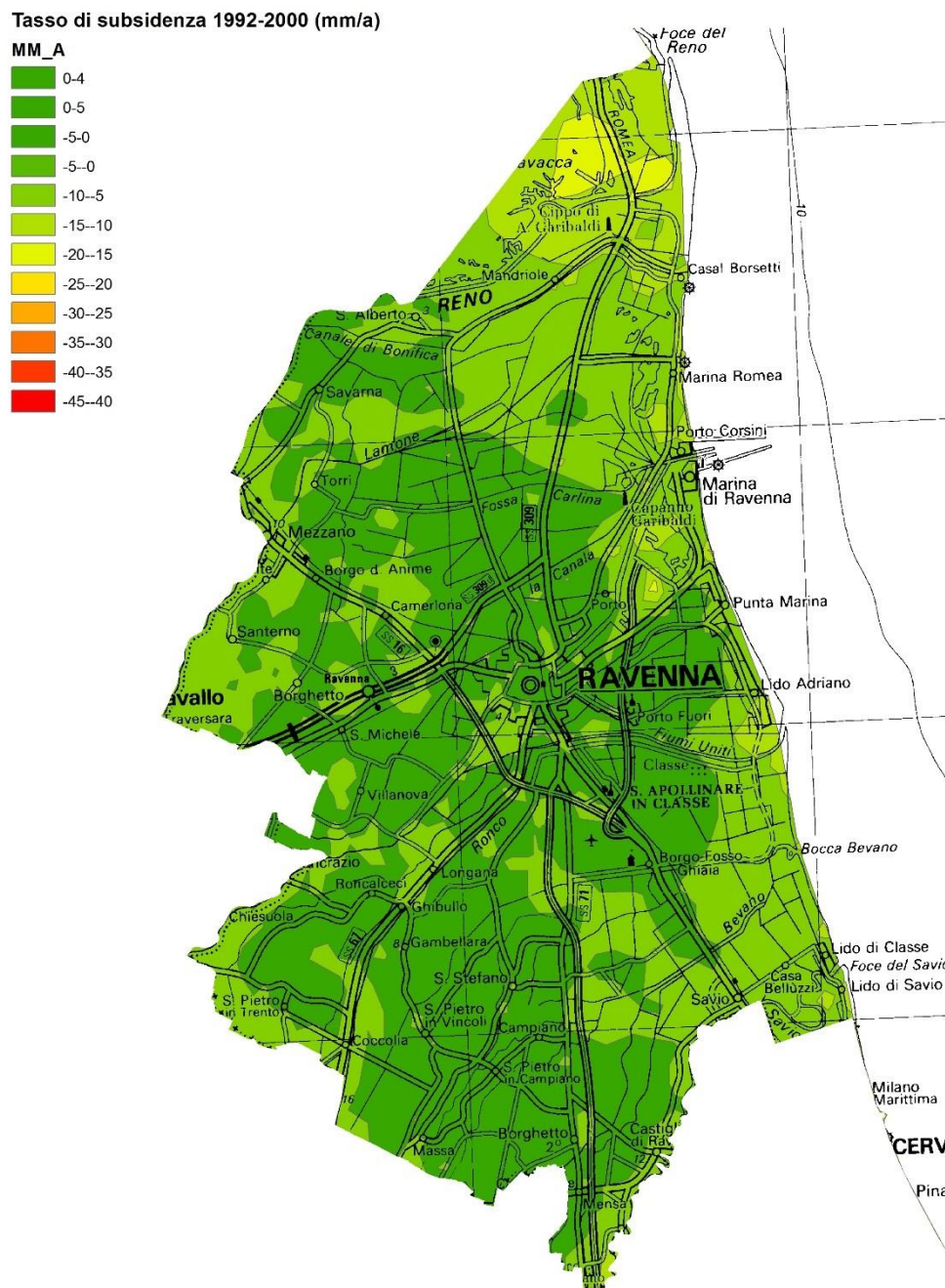
Fig. 2.1 – Tasso di subsidenza nel periodo 1992-2000 nell'area del Comune di Ravenna (Fonte ARPAE)
