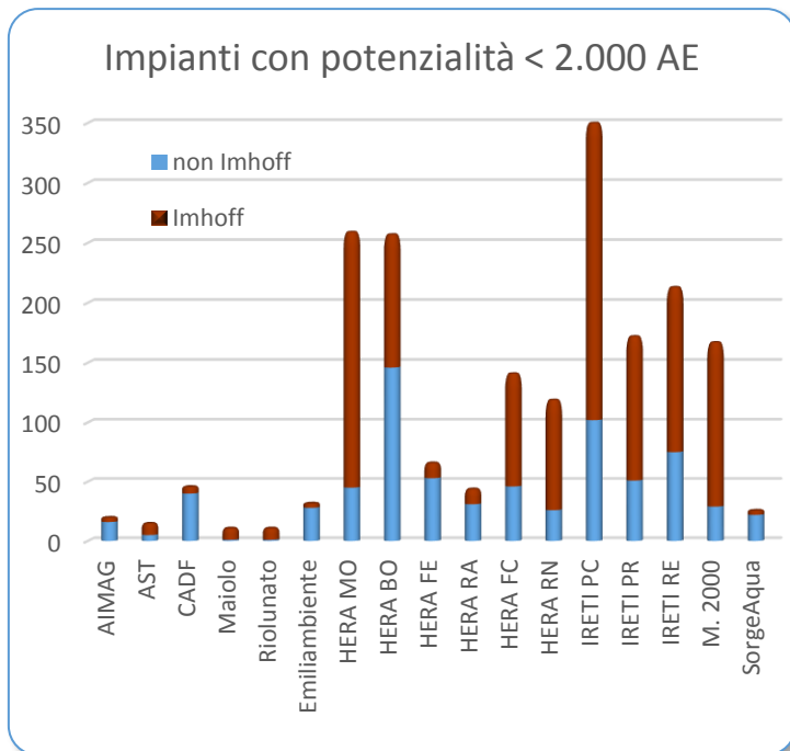
Grafico 11 – In numero di impianti di depurazione per gestore – dati 2017
