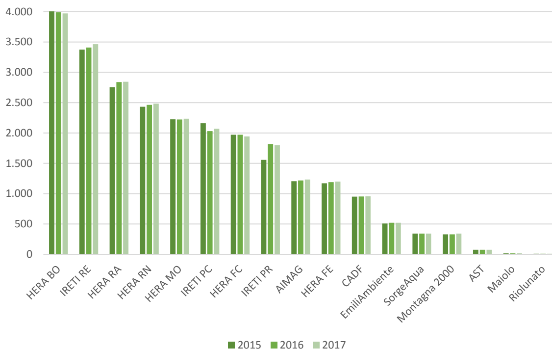
Lunghezza in km delle reti di fognatura
