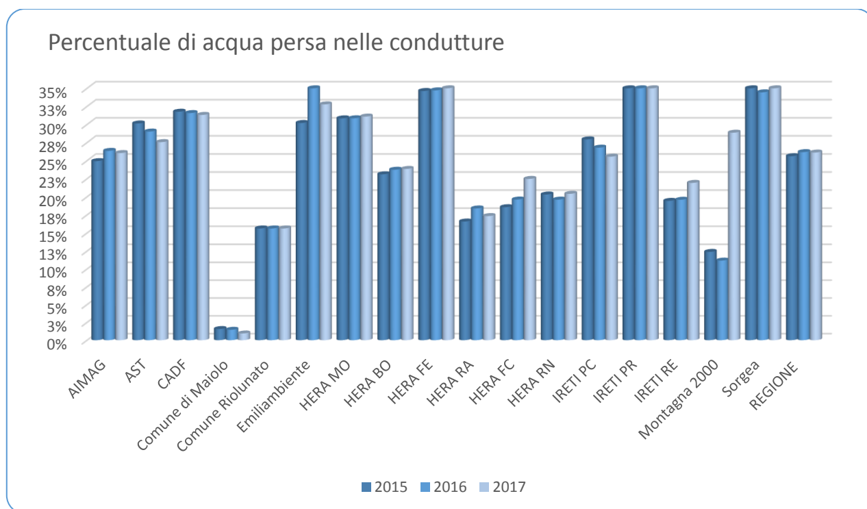
Grafico 5 - Il sistema di distribuzione dell'acqua potabile: le percentuali di acqua persa nelle condutture – 2015-2017
