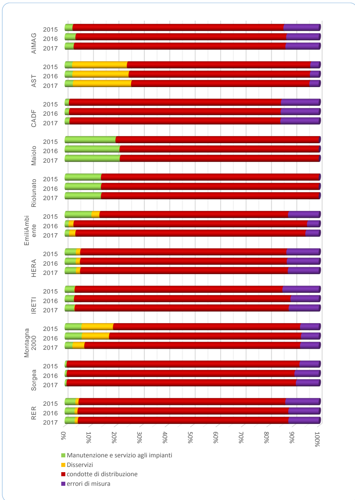
Grafico 4 - Il sistema di distribuzione dell'acqua potabile: le tipologie di perdita del sistema di distribuzione – 2015-2017
