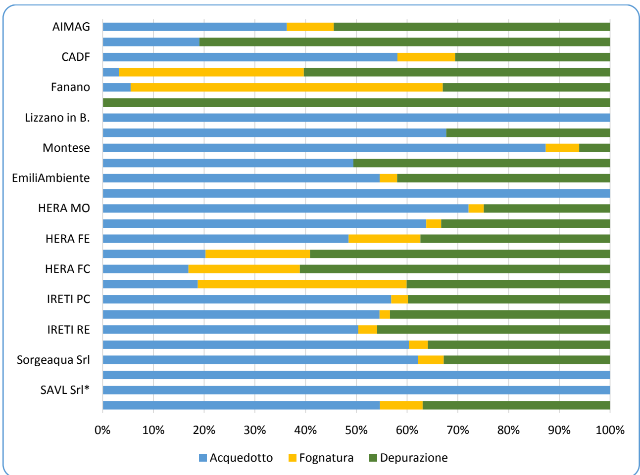
Grafico 12 - Rappresentazione dell'utilizzo di energia elettrica per segmento di servizio – dati 2018
