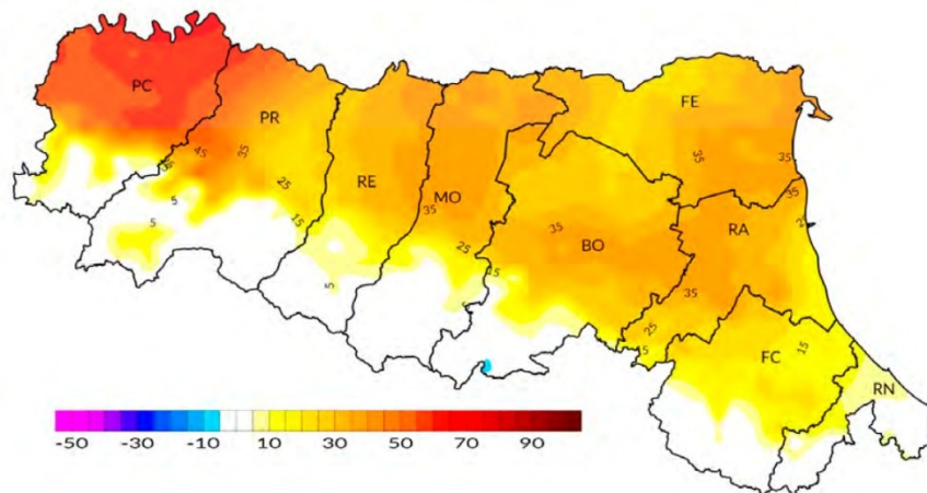
Fig. 3 - anomalia del numero di giorni caldi 2018 rispetto al clima 1961-1990
