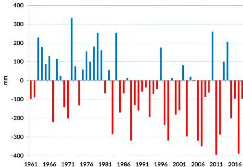
Fig. 5 - andamento temporale della media regionale del bilancio idroclimatico
