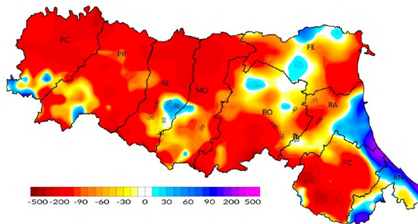
Fig. 4 - anomalia del bilancio idroclimatico annuo 2018 (mm) rispetto al clima 1961-1990
