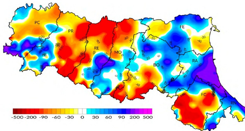
Fig. 2 – anomalia delle precipitazioni totali 2018 (mm) rispetto al clima 1961-1990
