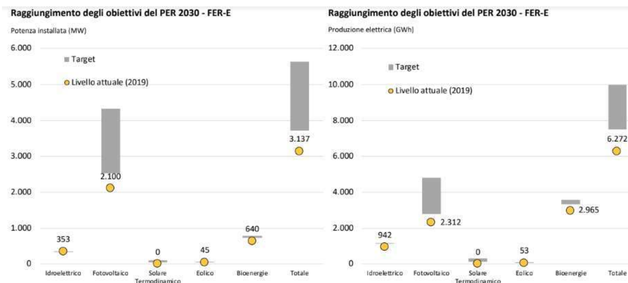
Figura 8-39> Raffronto Potenza e Produzione elettrica da FER in raffronto allo scenario del PER
