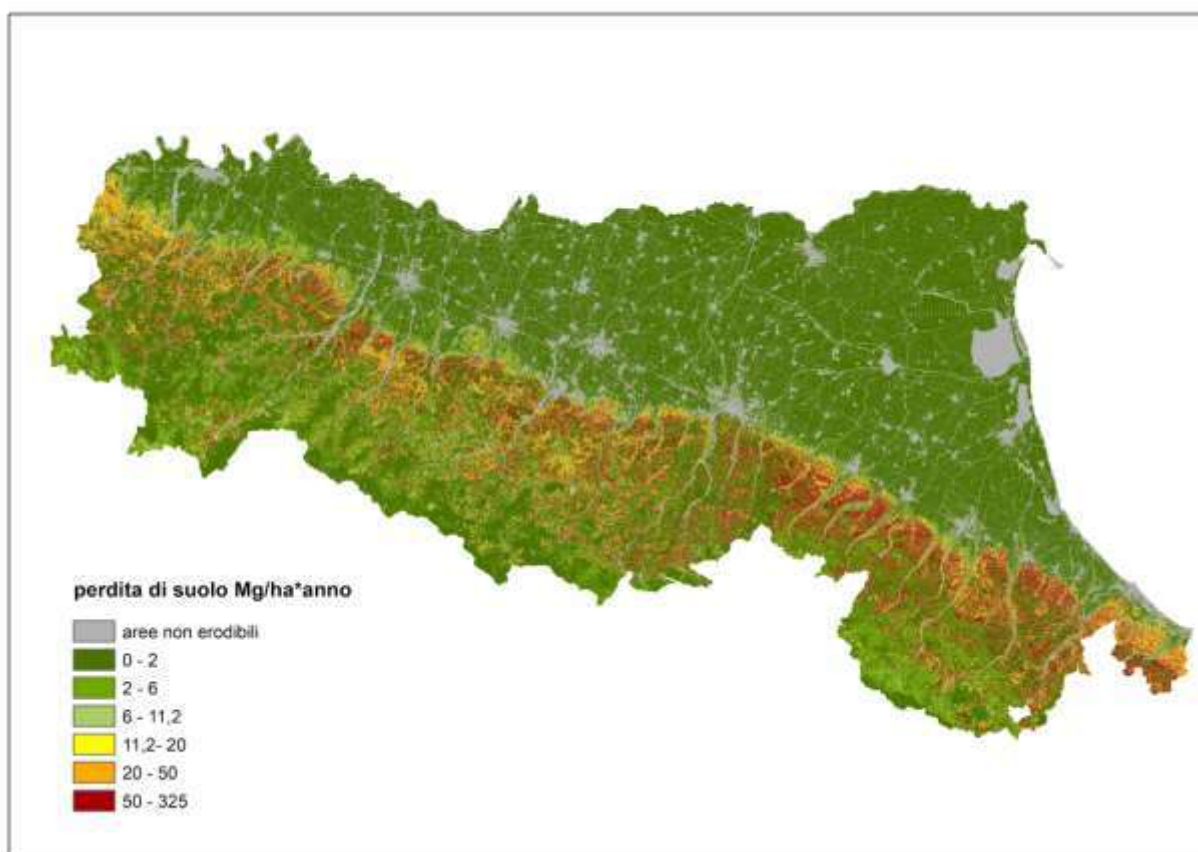
Figura 8-22> Carta erosione idrica attuale dei suoli dell'Emilia-Romagna, anno 2017
