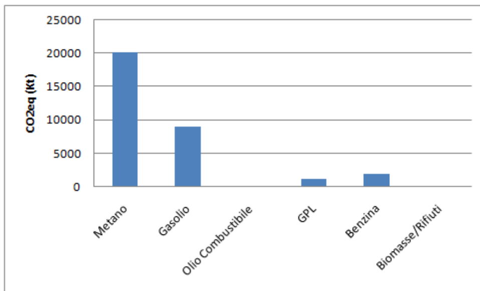
Figura 8-14> Emissioni CO 2eq per vettore energetico - Anno 2018
