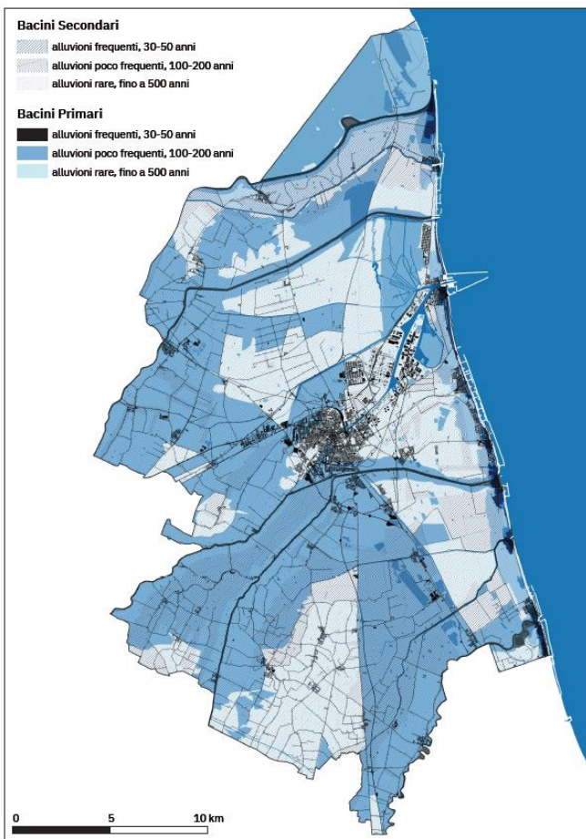
RISCHIO IDRAULICO
