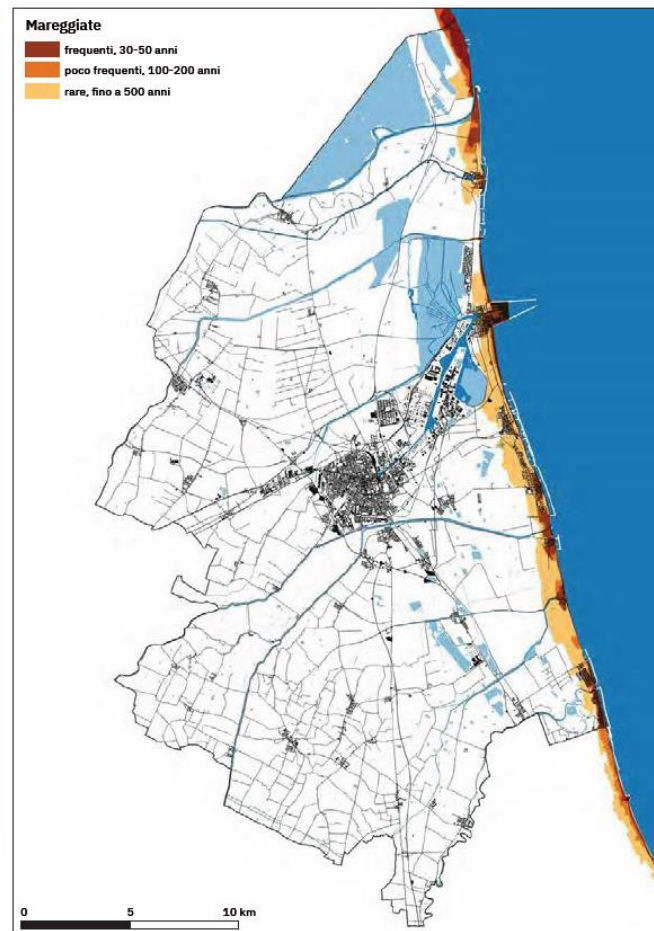
INGRESSIONE MARINA
