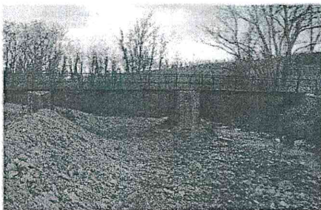
Posizionati gabbioni metallici per creare una briglia di contenimento
