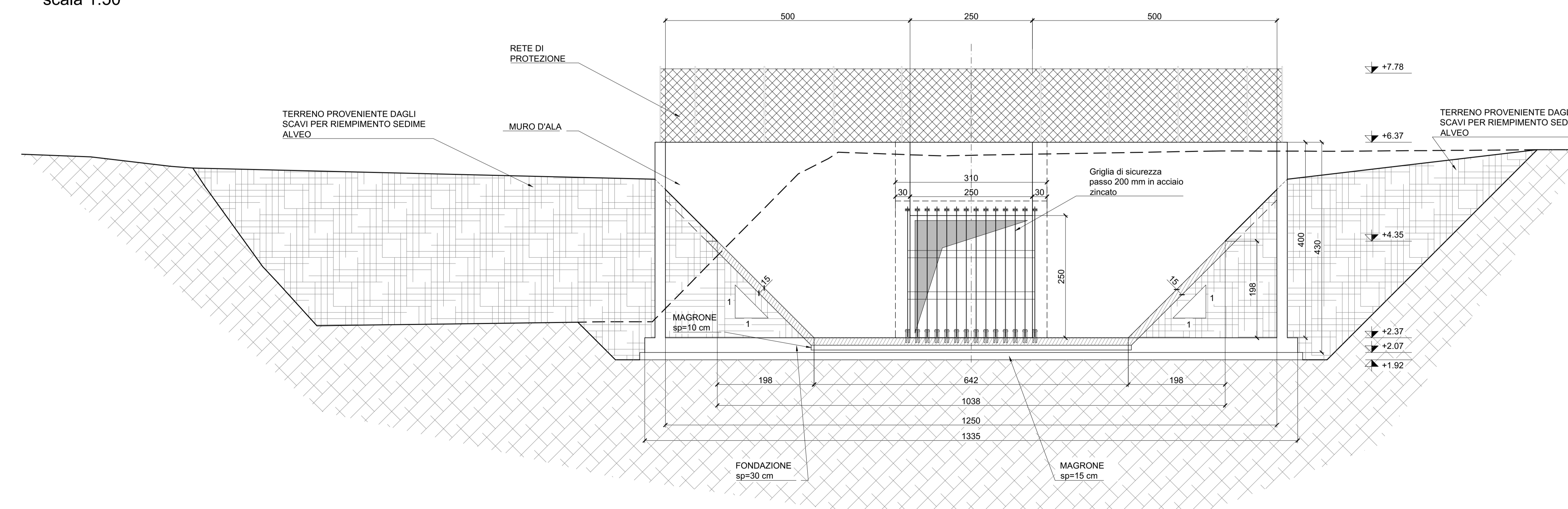
SEZIONE C-C scala 1:50
