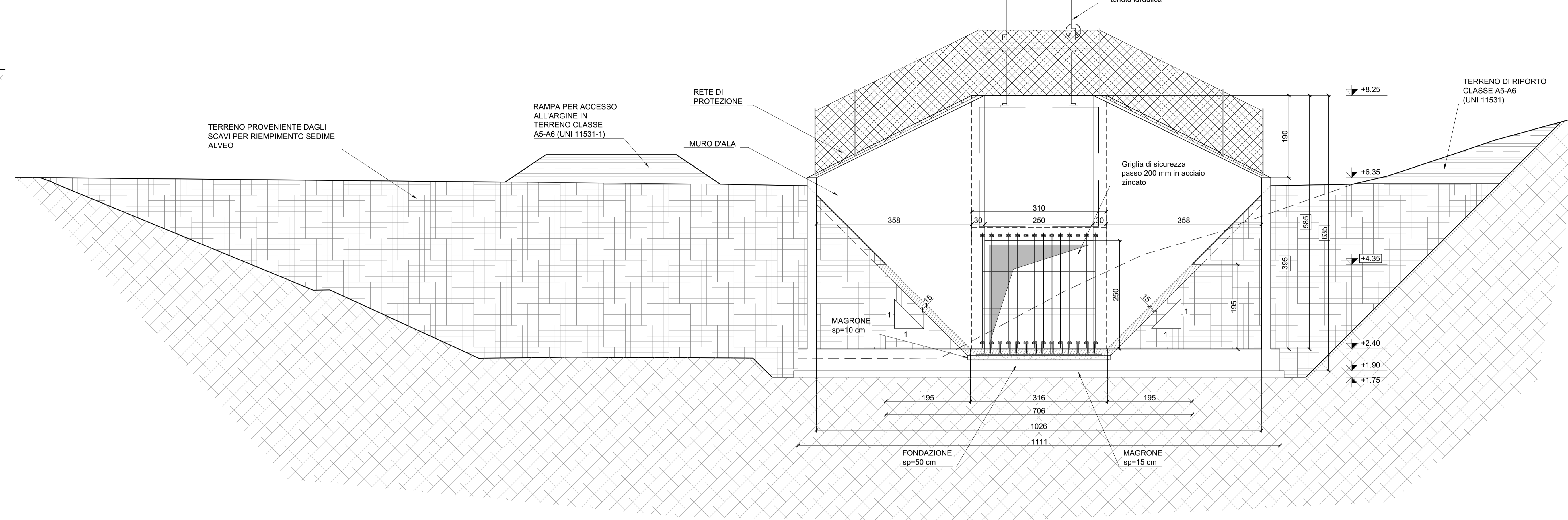
SEZIONE C-C scala 1:50
