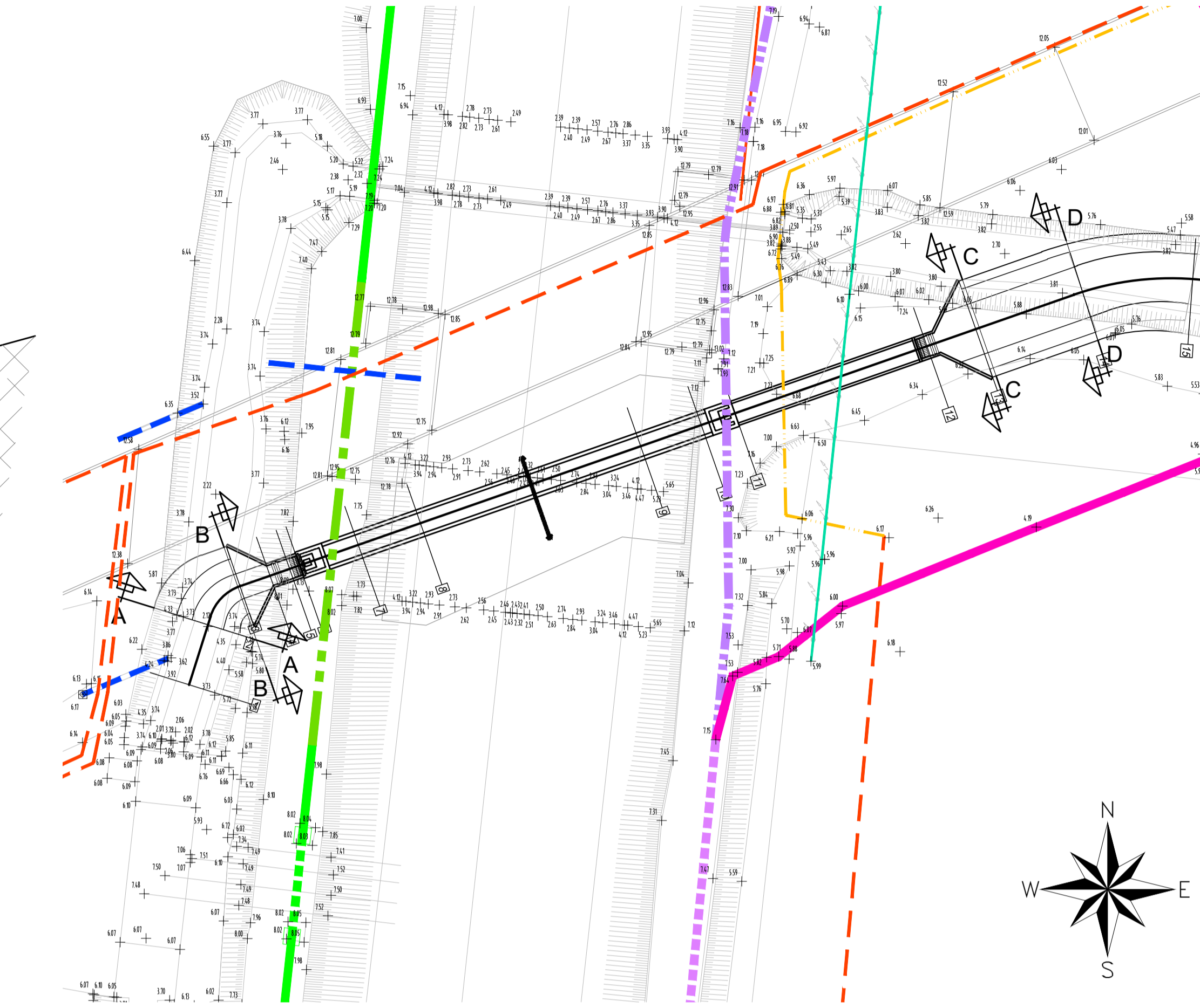
PLANIMETRIA SCALA 1:500
