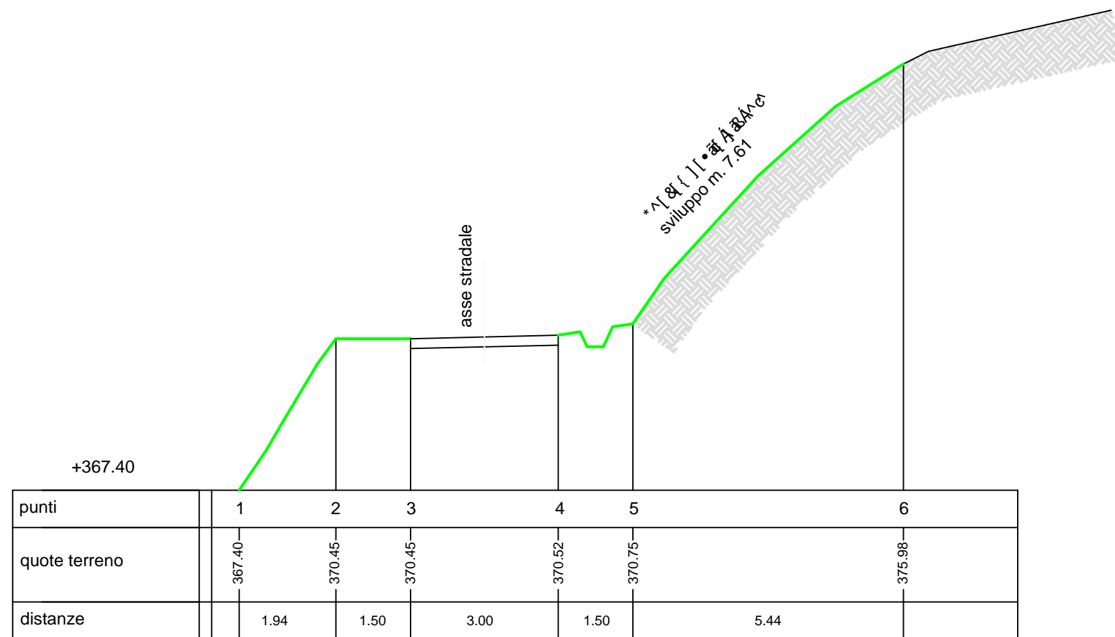
SEZIONE D 1:100
